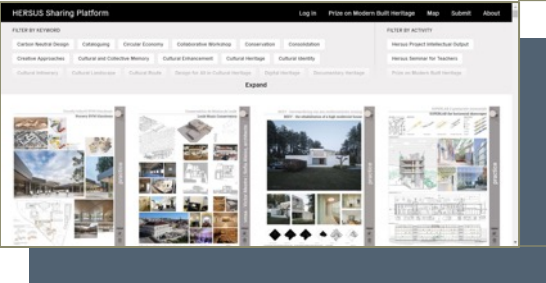
IO4 framework
